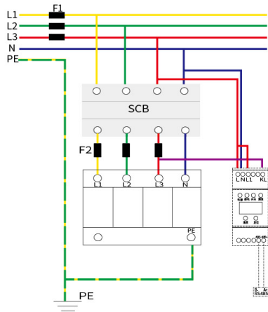
单模拼装接线图
