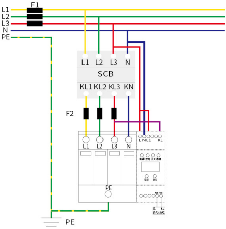
一体式接线图
